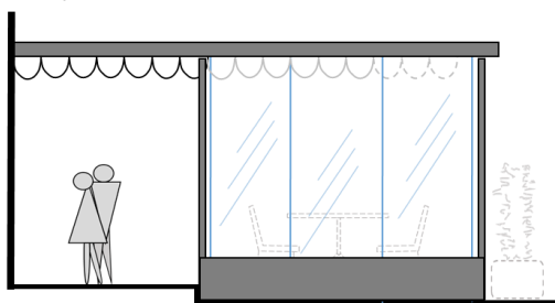
Prospetto laterale
